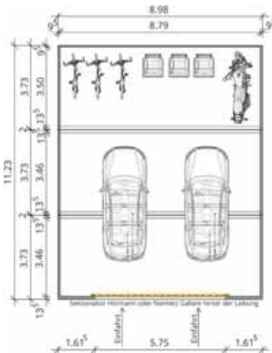
*Zeichnung links: Beispiel für 3 Garagenmodule hintereinander ohne Wandscheiben und Pfeiler. Auch unterschiedliche Längen sind kombinierbar. Mögliche Breiten der einzelnen Garagen: 5,98/ 6,48/ 7,48/ 8,48/ 8,98 m. Mögliche Längen der einzelnen Garagen: 2,73/ 2,98/ 3,23/ 3,48/ 3,73 m.
